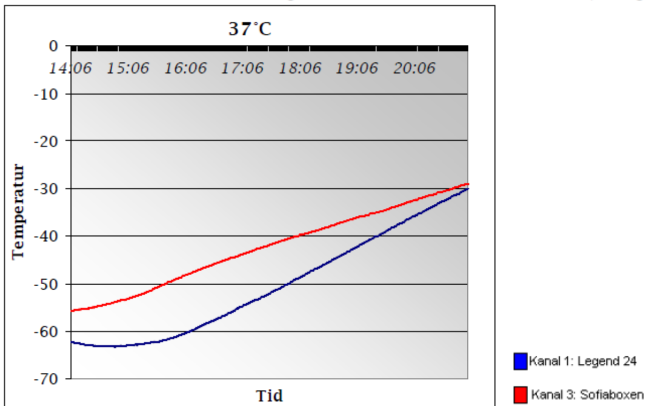
Diagram 4: Testning 4, 37°C, Kolsyreis
