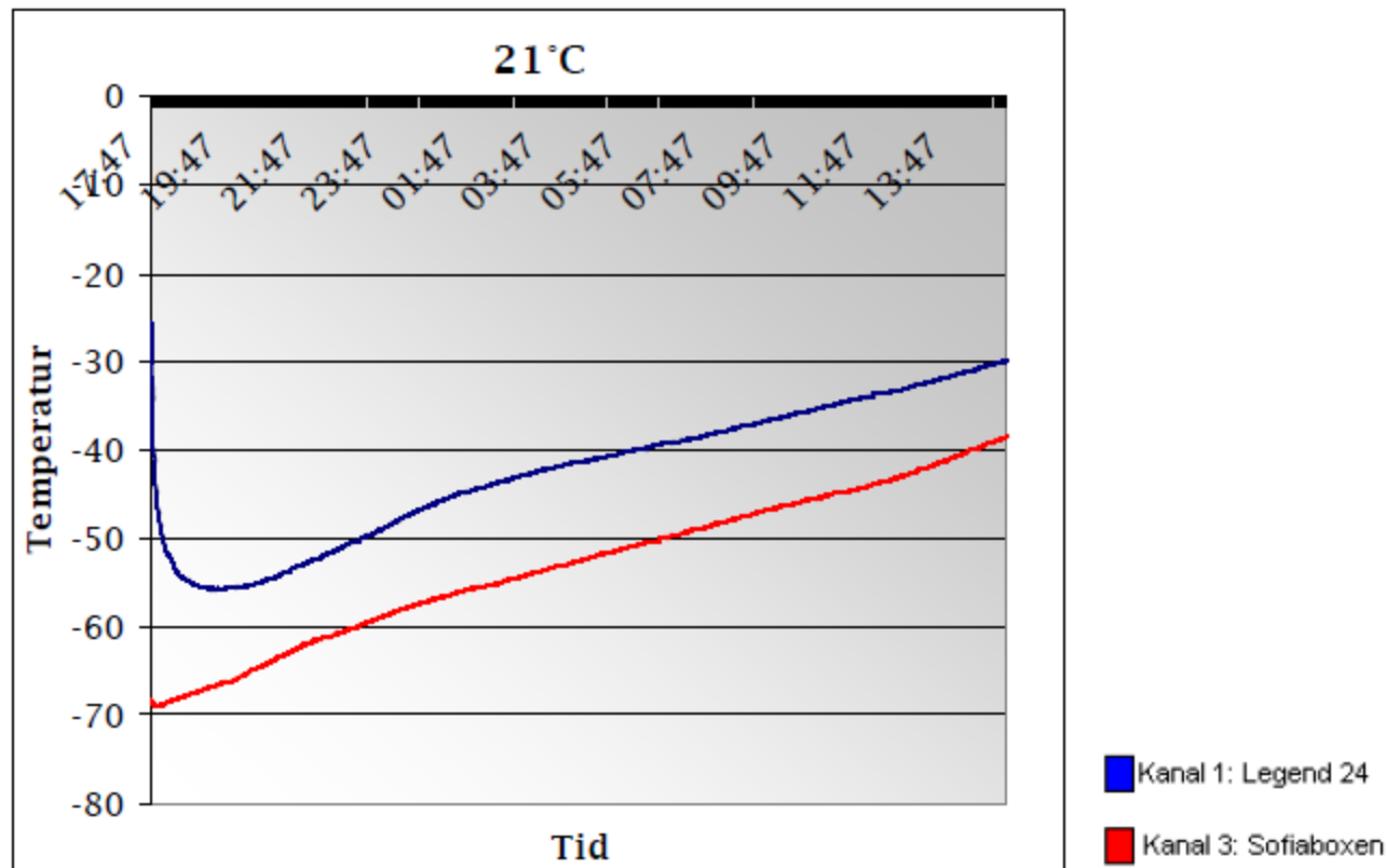
Diagram 3: Testning 3, 21°C, Kolsyreis
